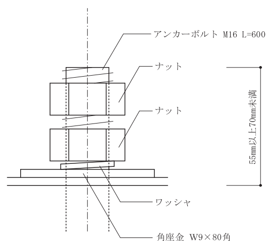
アンカーボルト突出部詳細
