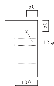
③ドリフトピン用穴あけ
