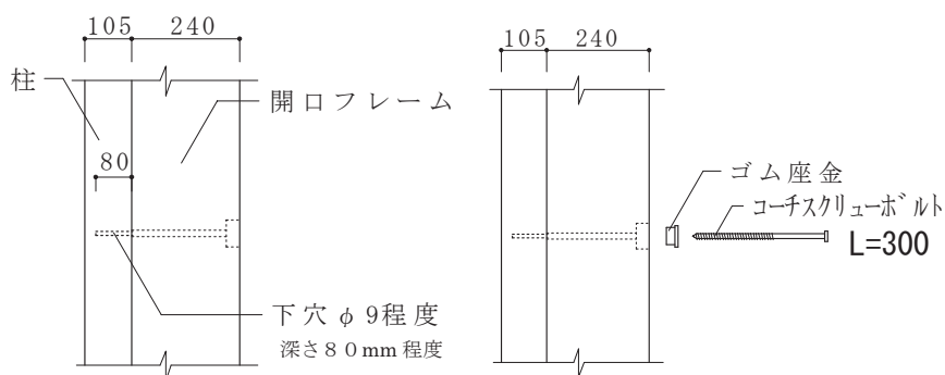
①柱・梁材への穴あけ
