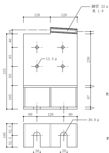
柱脚金物
