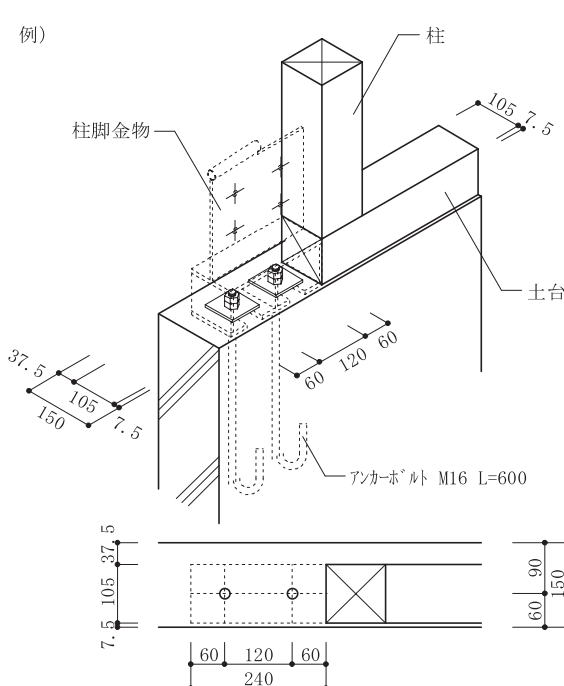
<基礎幅 150、土台 105×105 の場合>
